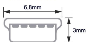
USB MINI B
