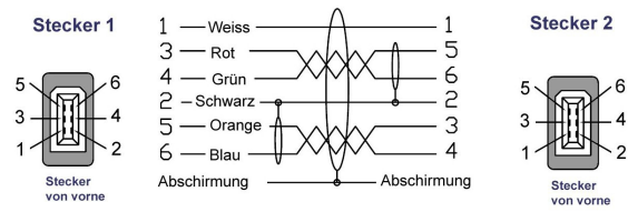
Pinbelegung 6-auf-6 Firewire
