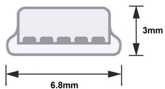
USB 2.0 Mini B
