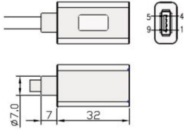
USB 3.0 A femelle
