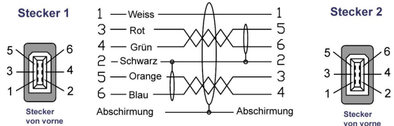
Pinbelegung 6-auf-6 Firewire
